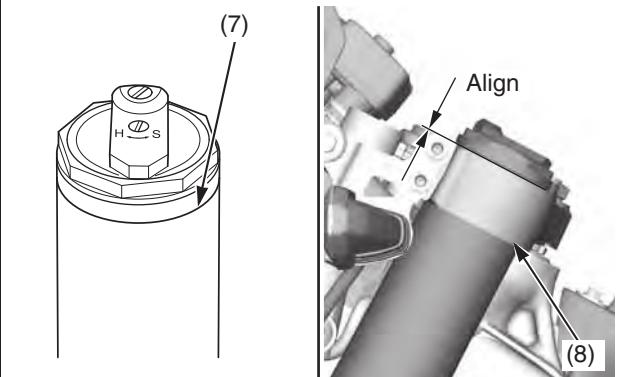
(7) groove
