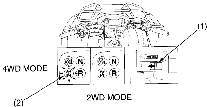
(2) 4WD indicator
