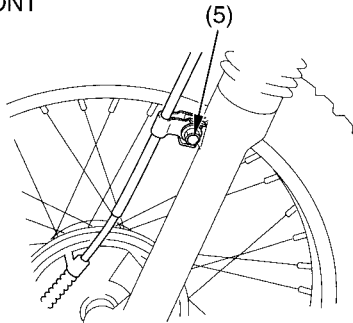
(5) cable guide bolt
